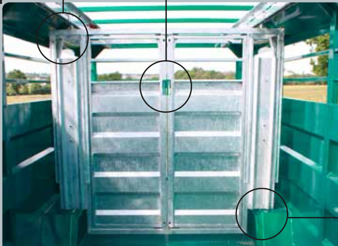
Schiebetrennwand mit zwei Türen
